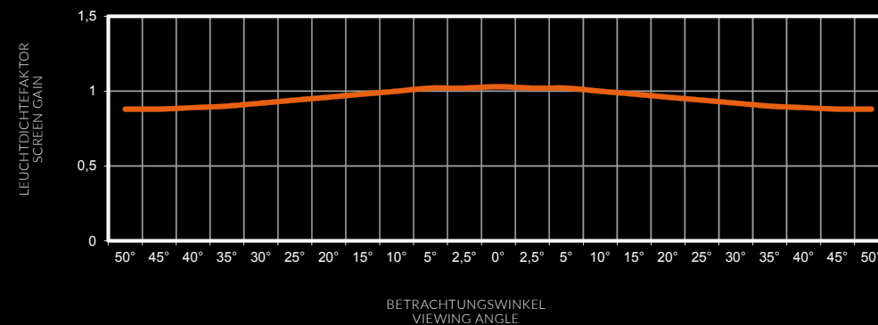
LEUCHTDICHTEFAKTOR NACH DIN 19045 | GAIN ACCORDING TO DIN 19045
